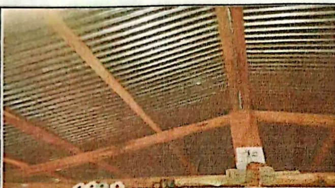
Foto 3: Sustitucion de Vigas y Costaneras.
